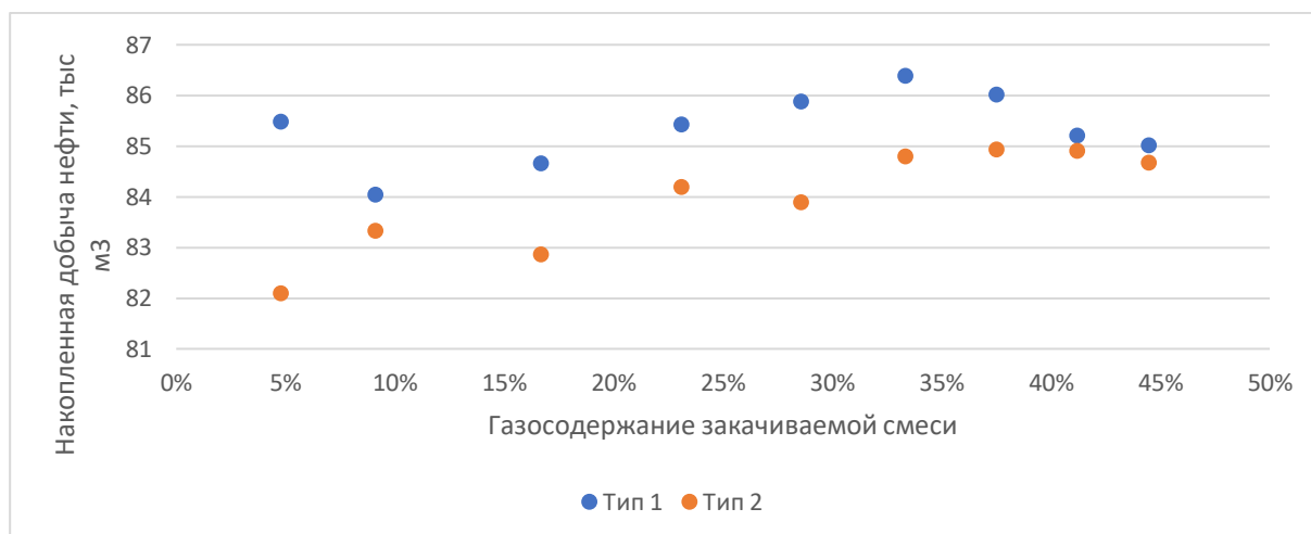
Рисунок 3 — Накопленная добыча для разнородных пластов в случае стационарного ВГВ
