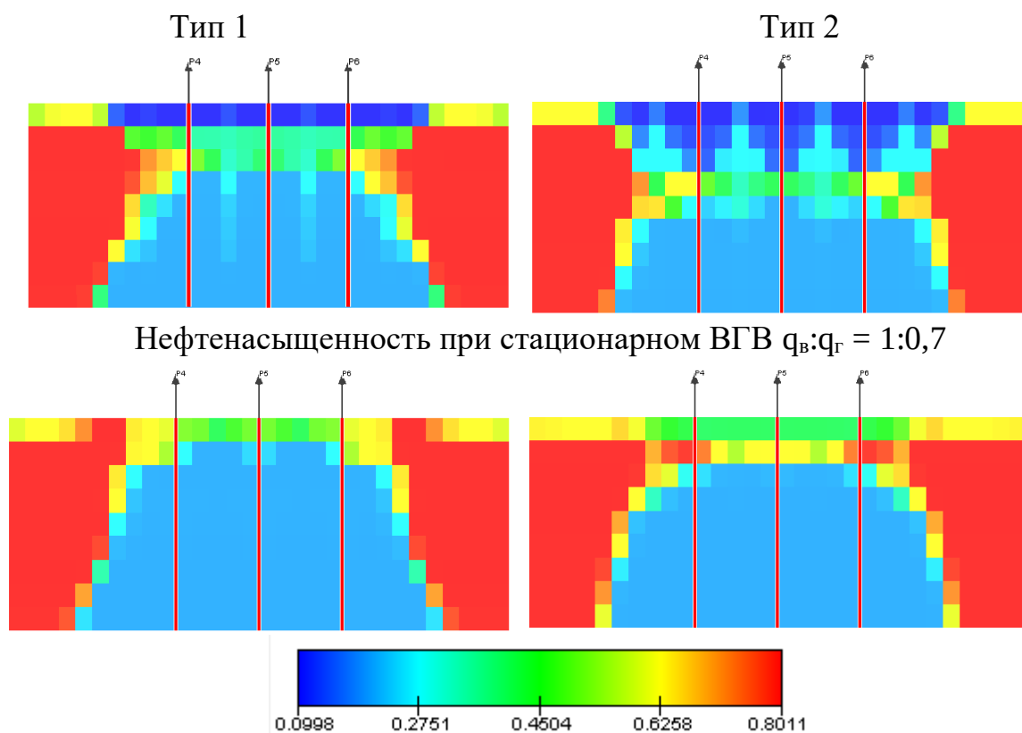
Нефтенасыщенность при нестационарном ВГВ В10:Г1 Рисунок 6 — Распределение остаточной нефтенасыщенности
