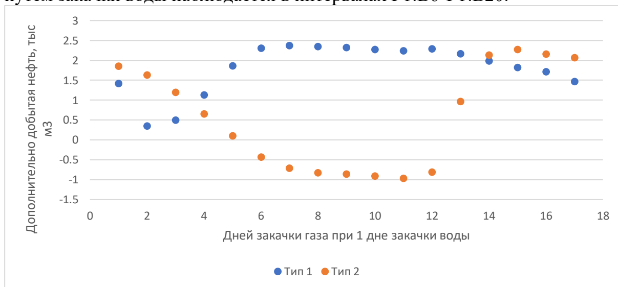
Рисунок 5 — Эффект применения нестационарного ВГВ
