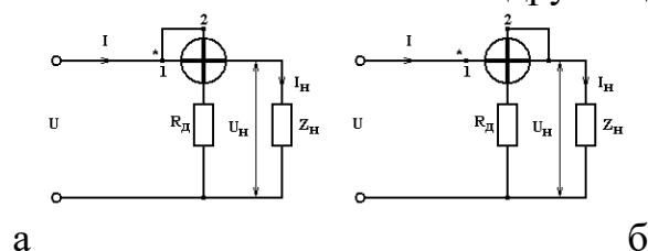
Рисунок 3 – Ваттметры на основе электродинамического преобразователя
