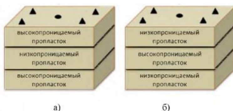
Рисунок 1 — Типы проницаемостной неоднородности
