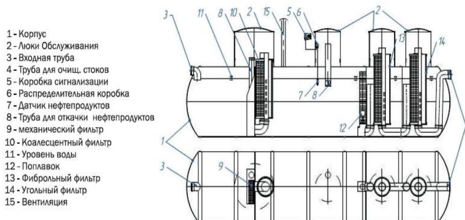
Рис. 1. Установка для очистки сточных вод
