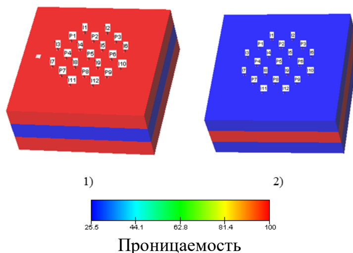
Рисунок 2 — Модели неоднородных пластов
