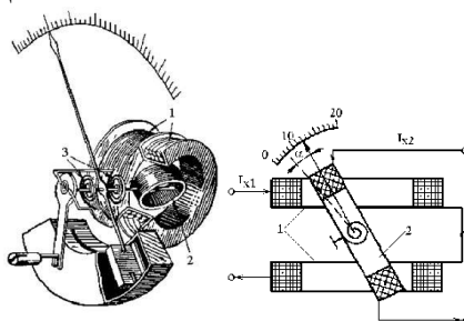
Рисунок 1 – Электродинамический преобразователь
