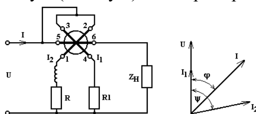
а- Электрическая схема фазометра б-векторная диаграмма фазометра Рисунок 4 – Фазометр на основе электродинамического преобразователя
