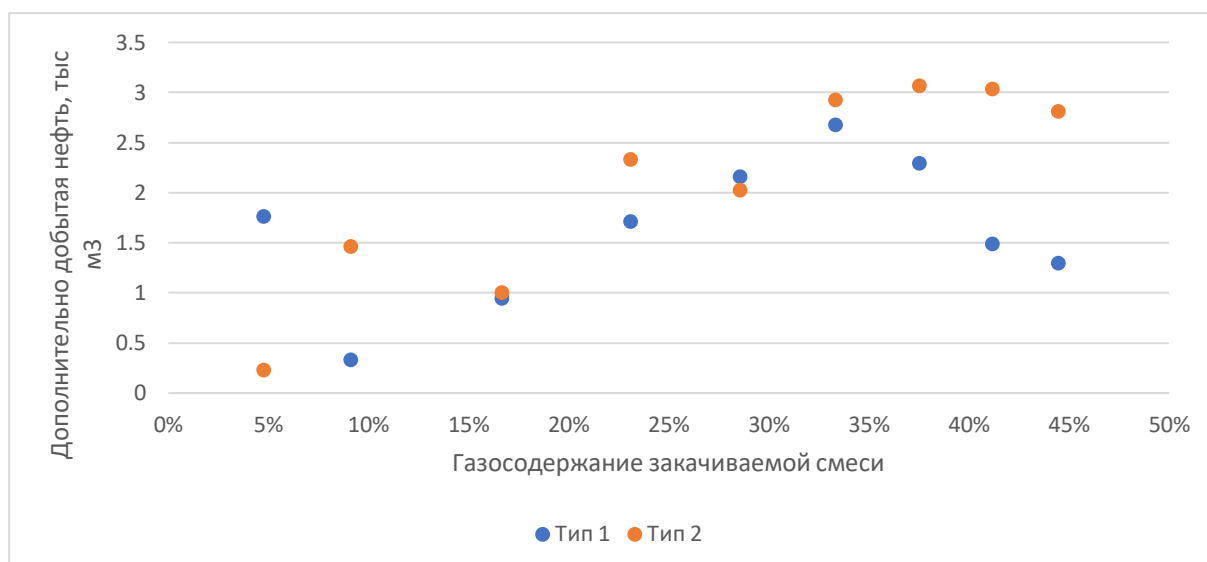
Рисунок 4 — Дополнительно добытое количество нефти
