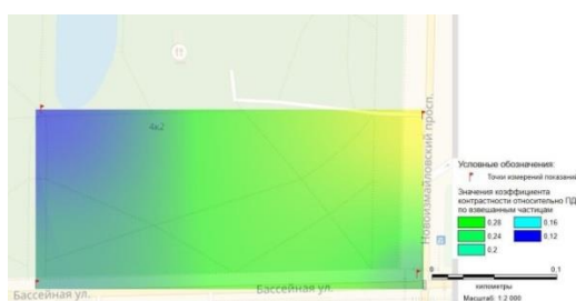
Рисунок 1 – Графические результаты мониторинговых исследований атмосферного воздуха парка Авиаторов г. Санкт-Петербург: а – CO, б – SO 2 , в – пыль неорганическая
