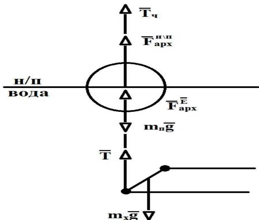
Рис.2. Распределение сил
