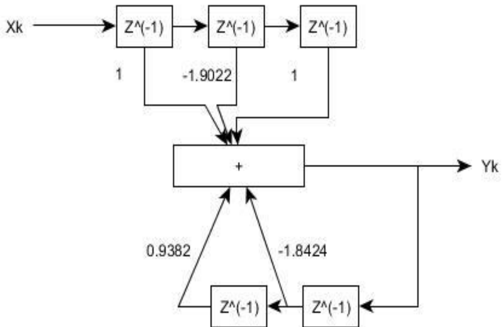
Рисунок 2 – Схема заграждающего фильтра
