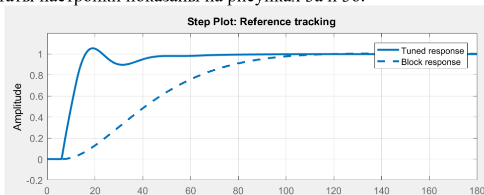
Рис 3а. Настройка ПИД-регулятора
