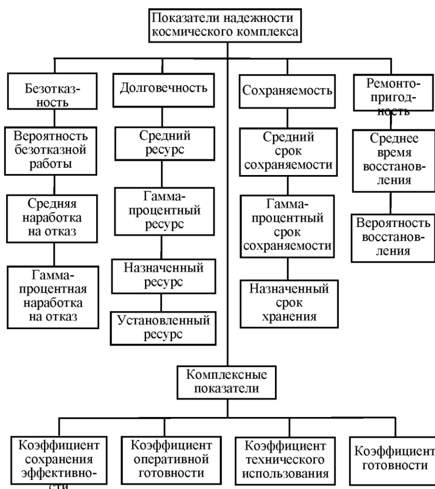
Рисунок 1 – Структура показателей надежности телеметрической аппаратуры
