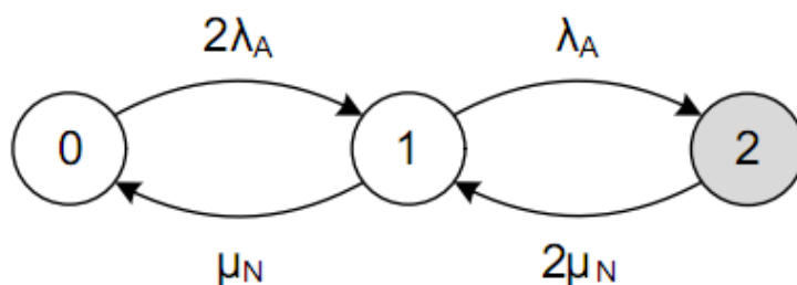
Рисунок 3 – Упрощенная модель надежности дублированной системы
