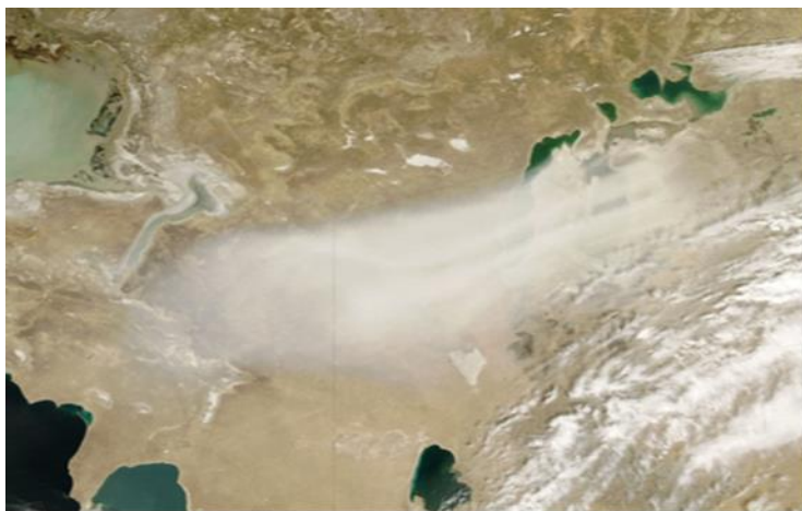
Рис.18. Ветровой вынос солей, синтезированное (1-3-ий каналы) изображение со спутника NOAA-19 ( www.econews.uz )
