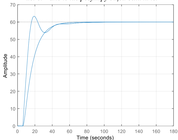
Рис. 7. Изменение регулируемой величины
