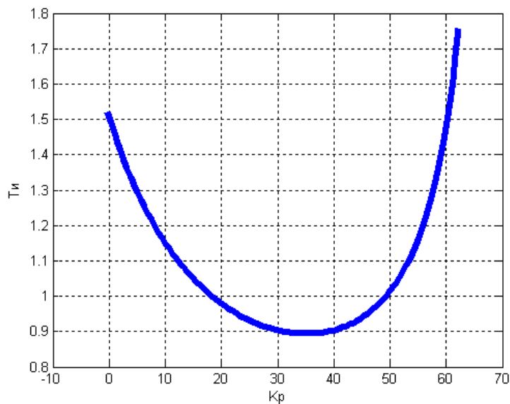
Рис. 1. разбиение в плоскости параметров ПИД-регулятора Расчёт и анализ системы управления
