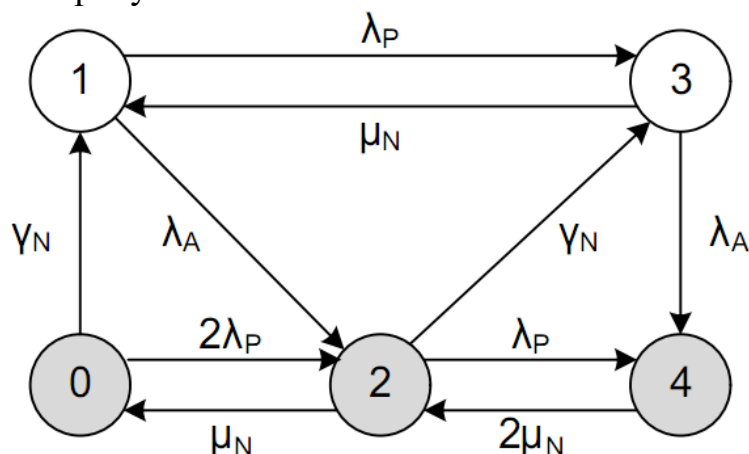
Рисунок 5 – Модель надежности систем с основным и резервным узлом
