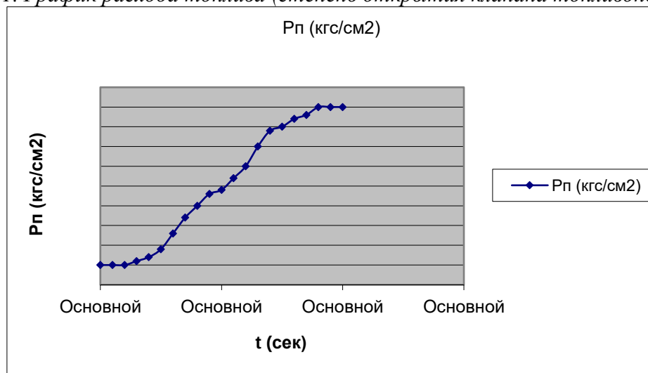
Рис. 2. Разгонная характеристика по каналу расход топлива - давление пара на выходе котла
