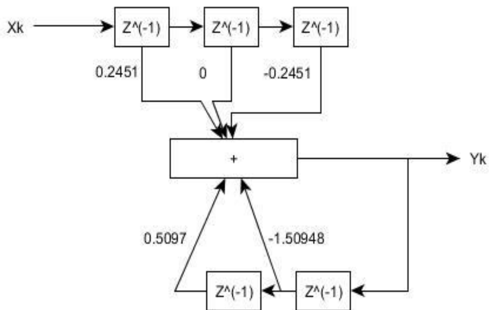
Рисунок 3 – Схема фильтра Баттерворта
