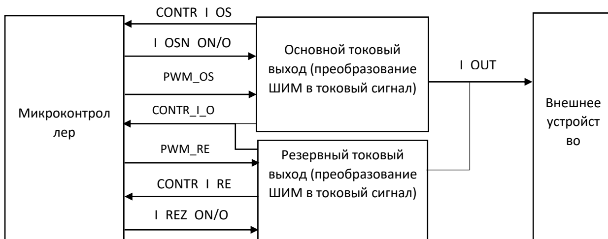
Рисунок 1 – Резервирование токового выхода газоанализатора
