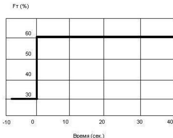
Рис. 1. График расхода топлива (степень открытия клапана топливоподачи)
