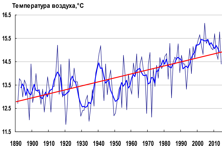
Рис. 1. Изменение среднегодовой температуры воздуха в Ташкенте. Тренд - 1.7 C/100 лет.
