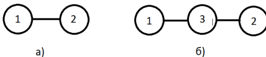
Рисунок 1 – Преобразование ребра \{1, 2\} в вершину 3
