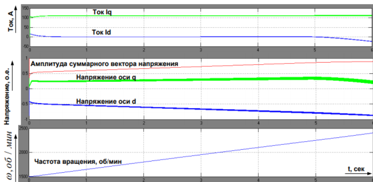
Рисунок 2. Разгон двигателя от 1500 об/мин до 2500 об/мин в условиях нехватки питающего напряжения
