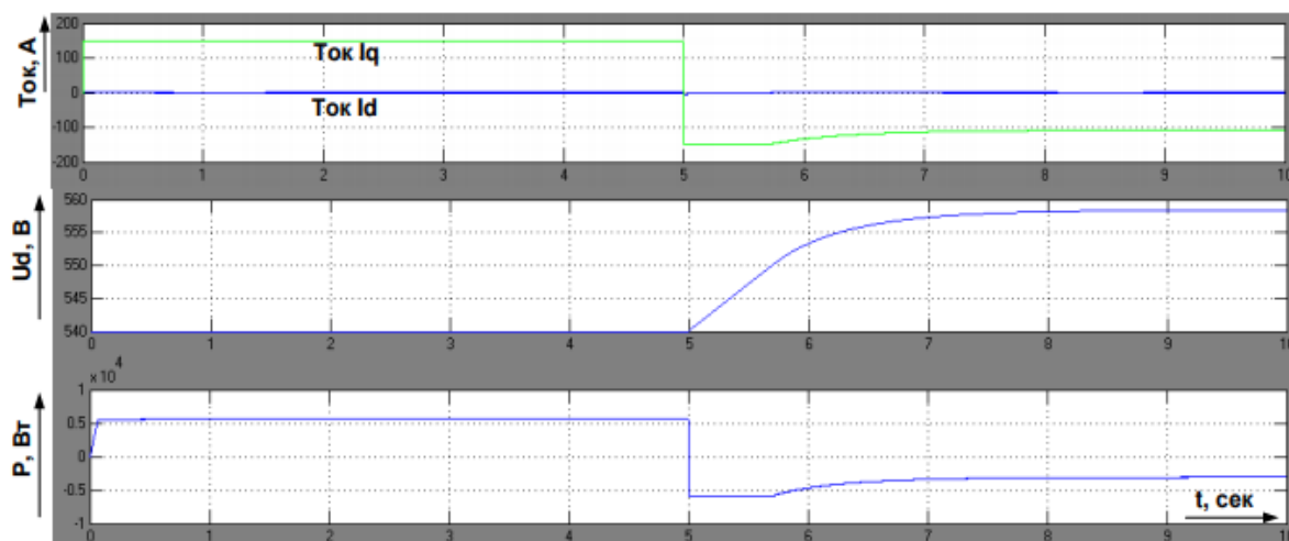
Рисунок 4. Смена двигательного режима на генераторный с последующей рекуперацией в звено постоянного тока
