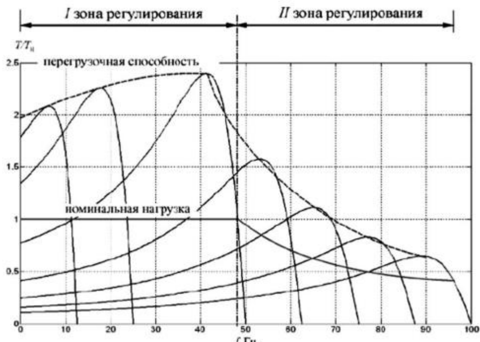
Рисунок 1 - Механические характеристики асинхронного двигателя, работающего в составе частотно-регулируемого электропривода
