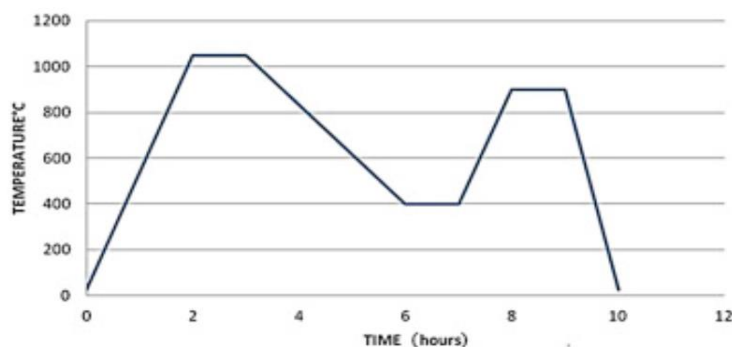
Рисунок 1. Цикл термообработки для разливки стали (вертикально указана температура, горизонтально время)
