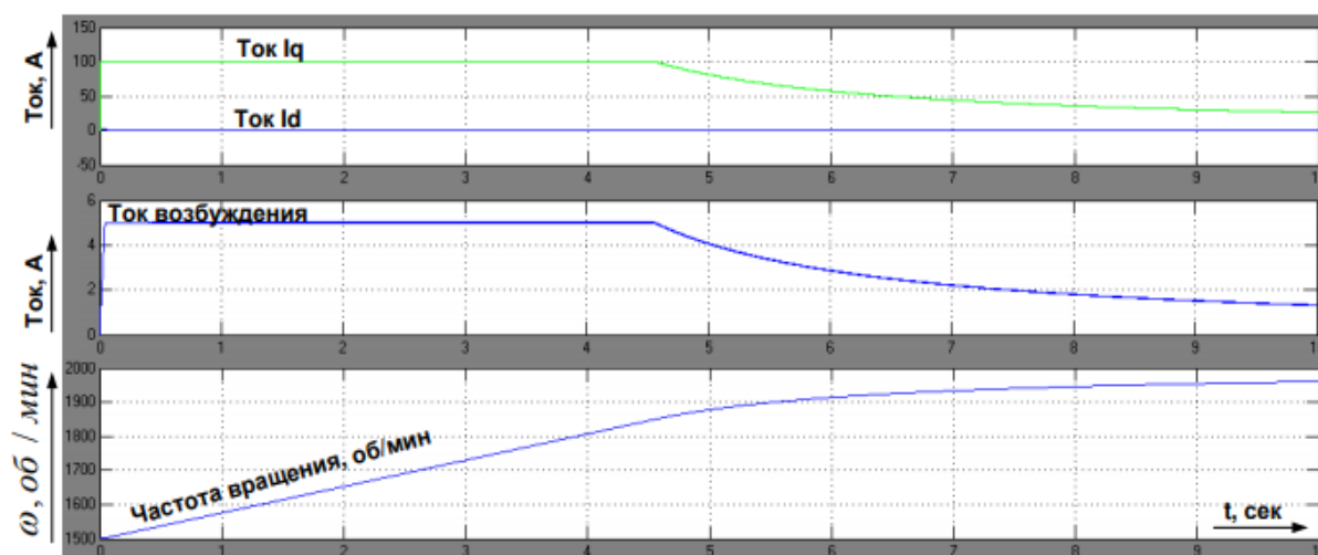
Рисунок 3. Разгон двигателя от 1500 об/мин до 2000 об/мин в условиях ограничения частоты вращения
