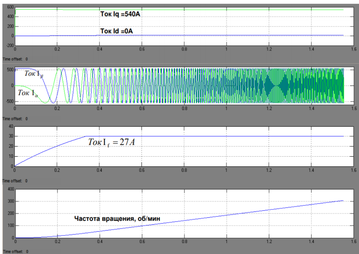
Рисунок 1. Разгон двигателя с нулевой частоты вращения до 300 об/мин с максимальным моментом
