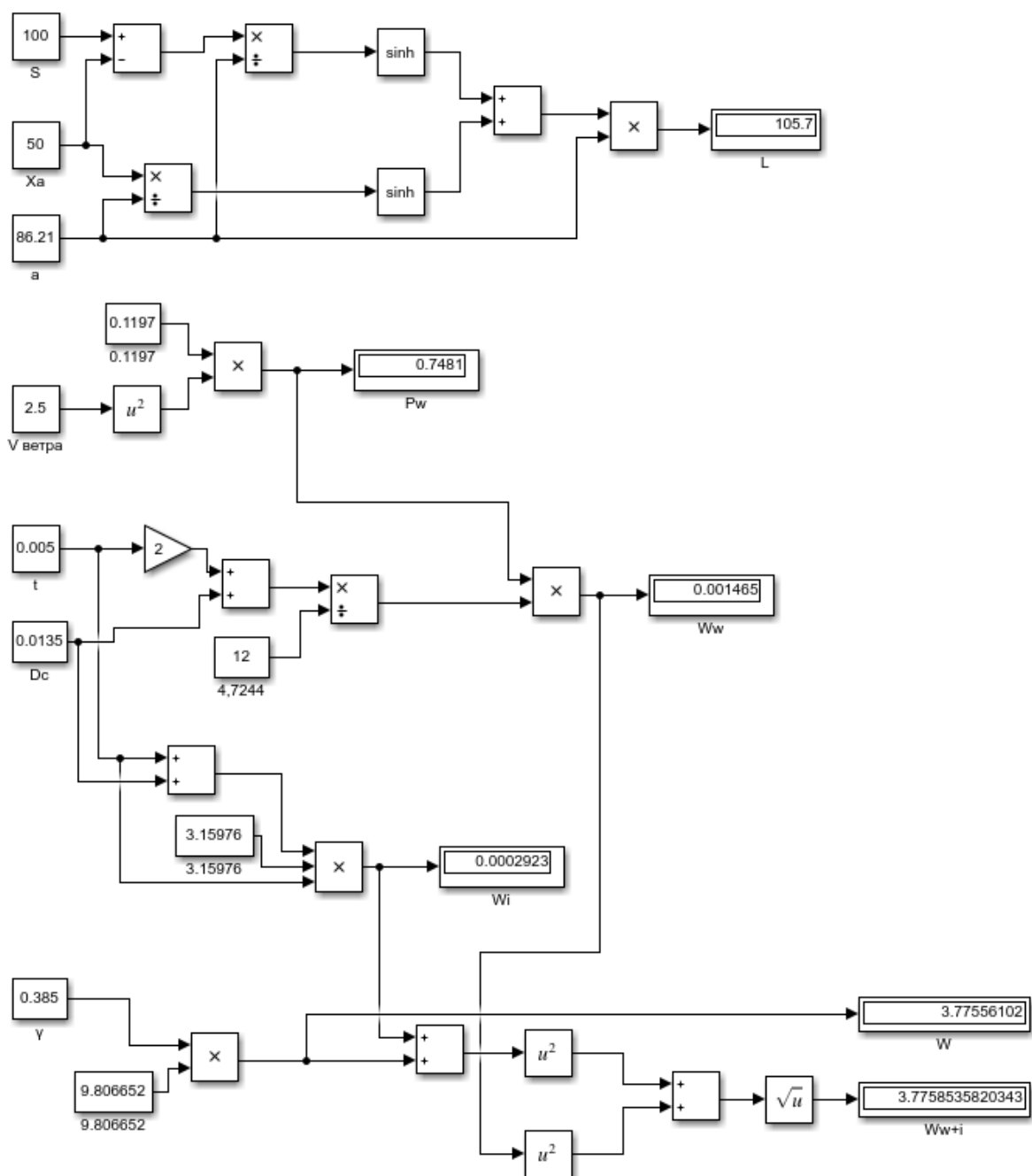
Рисунок 1 – Модель примера в пакете Matlab/Simulink
