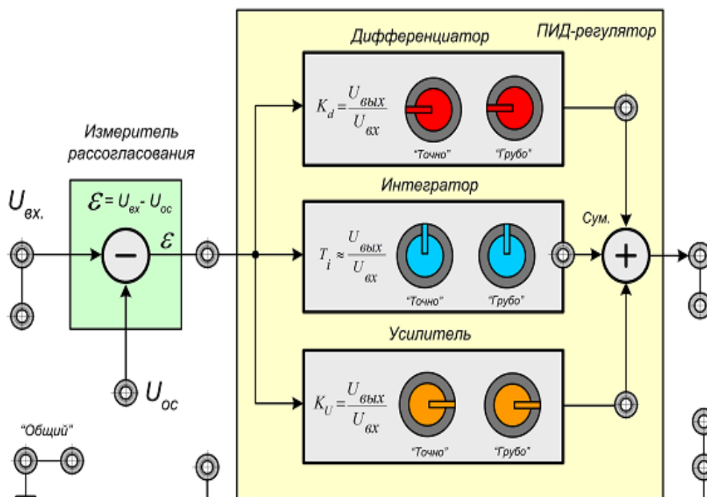
Рисунок 4. Панель управления «Измеритель рассогласования и ПИД-регулятора».
