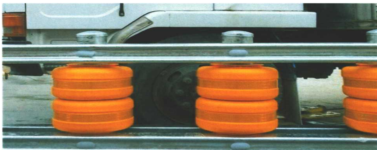
Рис. 2. Применение двух роликовых «крутящие» конструкции гибкого барьерного ограждения.
