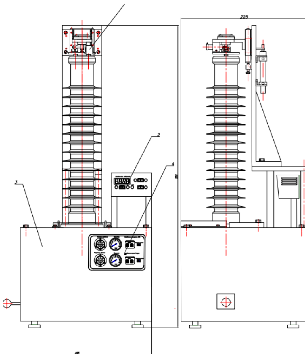
Рисунок 1- Устройство контроля положения ограничителей перенапряжения при установке верхнего терминала.
