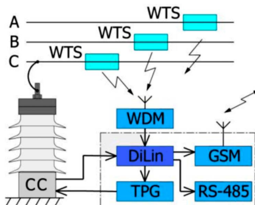
Рисунок 3 - Система DiLin на ЛЭП
