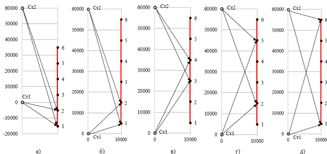
Рисунок 1 – Варианты взаиморасположения станций и связующих точек
