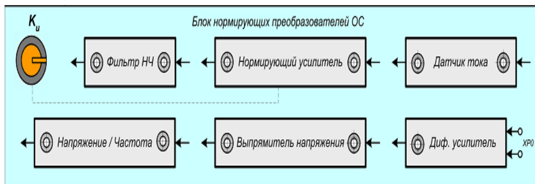
Рисунок 7. Панель управления «блока нормирующих преобразователей обратной связи».
