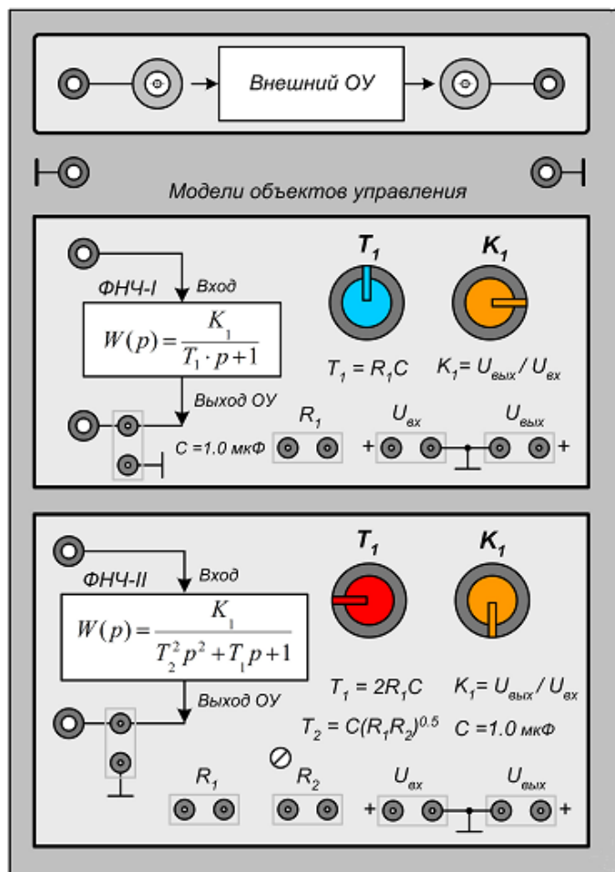
Рисунок 6. Панель управления «Модели объектов управления».
